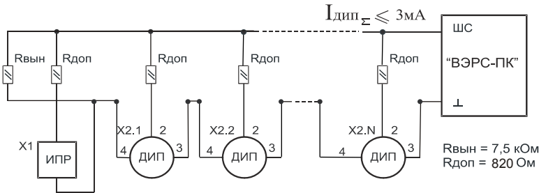
Рисунок.Б6. Схемы включения ШС типа ШНС и ШПНС с несколькими дымовыми извещателями (типа ИП212). Двухпороговый алгоритм с верификацией.
