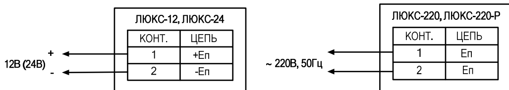
Рис.1. Схемы подключения.
