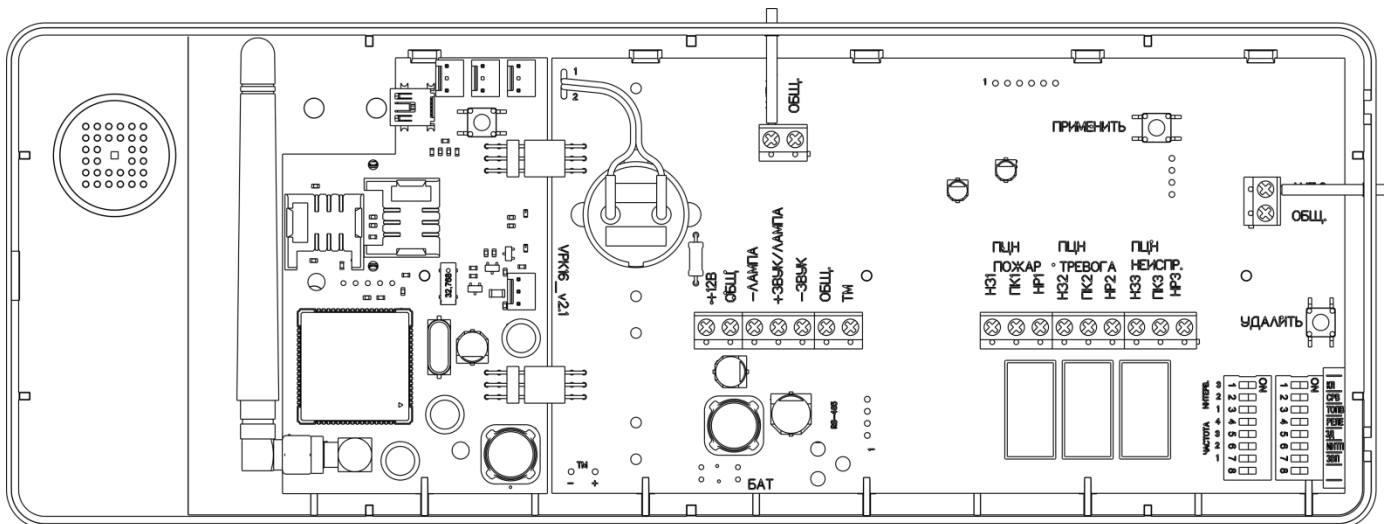
Рис.3. Внешний вид платы прибора ВС-ПК ВЕКТОР-АР GSM-100.
