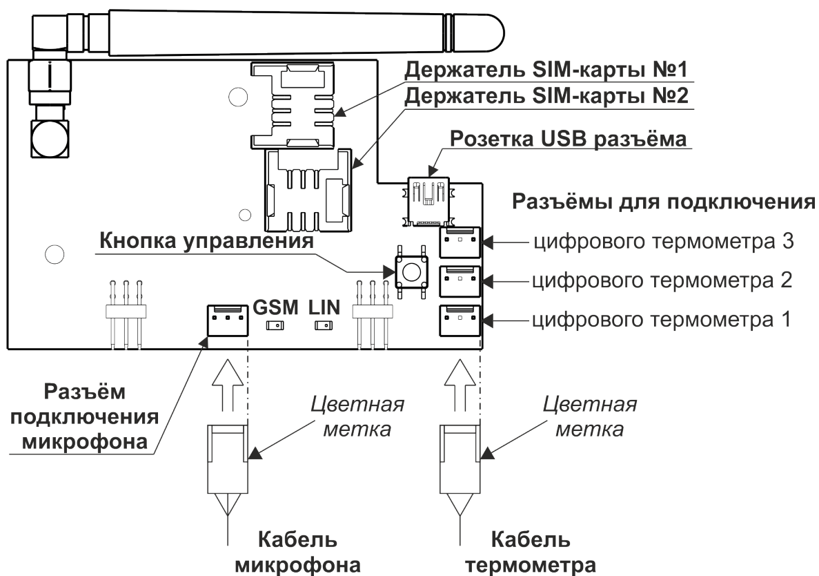
Рис.4. Внешний вид платы коммуникатора прибора ВС-ПК ВЕКТОР-АР GSM-100.
